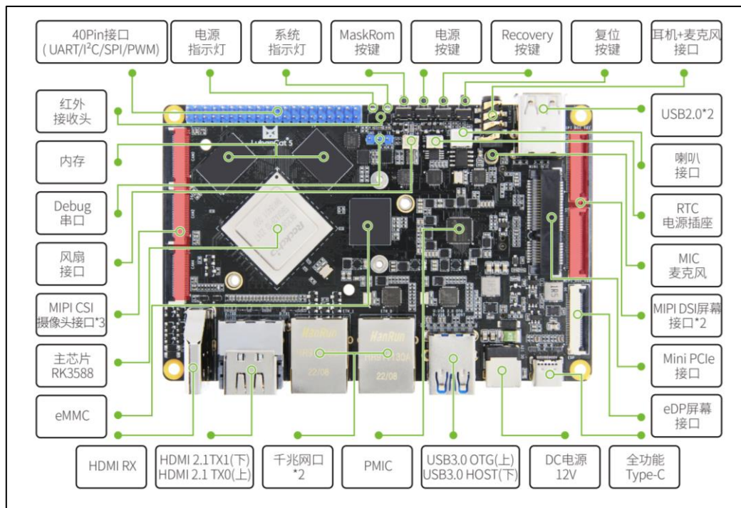
图 3.2.1-1 鲁班猫 5-V1 正面视图
