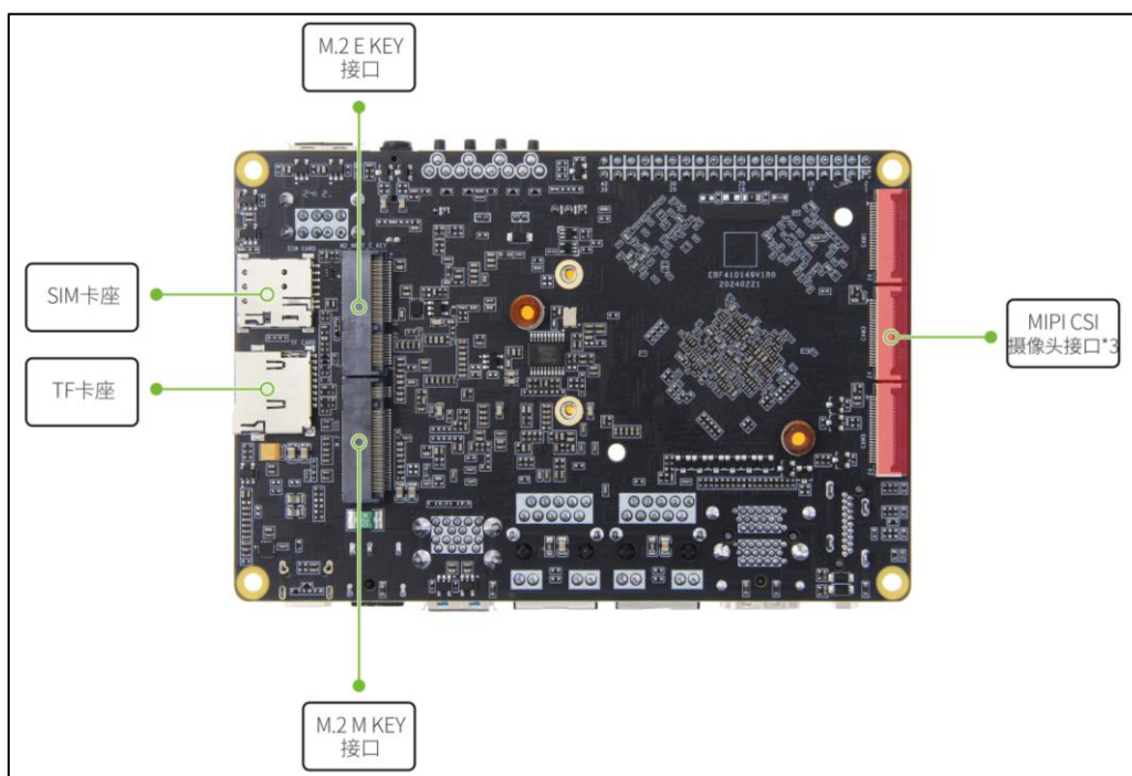
图 3.2.1-4 鲁班猫 5-V2 背面视图
